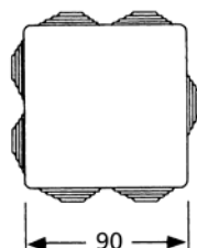
Ref. 604 7 conos para tubo de \varnothing 20 (M20).
