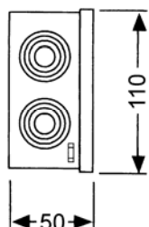
Ref. 615 7 conos para tubo de \varnothing 25 (M25).
