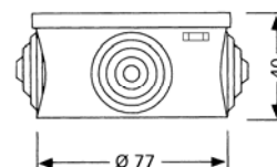
Ref. 665 4 conos para tubo de \varnothing 20 (M20).
